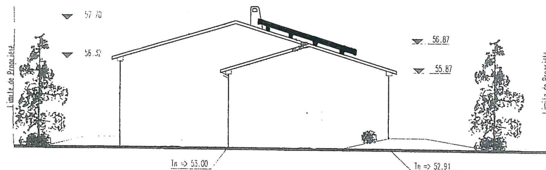
FACADE OUEST - 1/100 -
