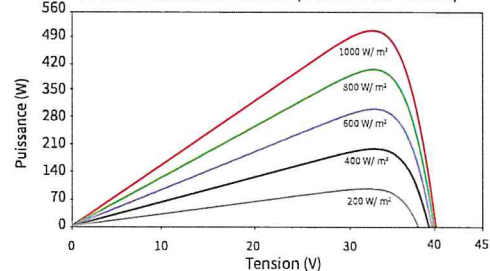
Courbe Puissance-Tension (54HL4M-BDV 505W)
